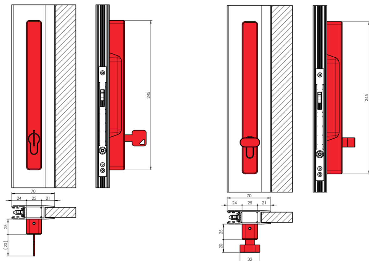
Griff mit Schloss, Betätigung mit einem Schlüssel
