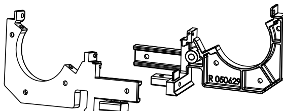
Verbindungskonsole LINKS/RECHTS (6-014687 / 6-014688)
