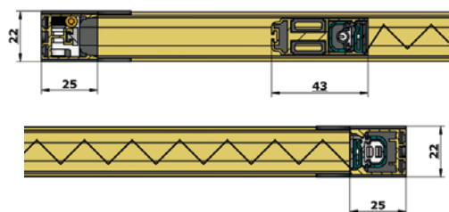
Horizontalschnitt
