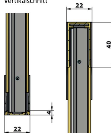
Vertikalschnitt
