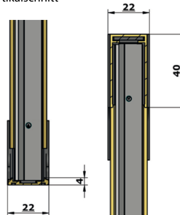
Vertikalschnitt
