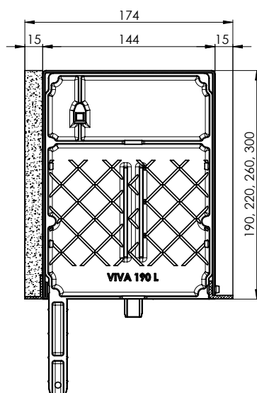
Schnitt durch den Unterputz-Kasten VIVA 190 x 160L2VP 220 x 160L2VP 260 x 160L2VP 300 x 160L2VP
