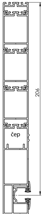
Größtmögliche Erweiterung des Grundprofils P 081
