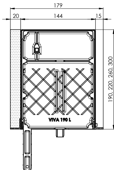
Schnitt durch den Unterputz-Kasten VIVA 190 x 179 x 2L x STY20 220 x 179 x 2L x STY20 260 x 179 x 2L x STY20 300 x 179 x 2L x STY20
