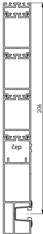
Größtmögliche Erweiterung des Grundprofils P 020
