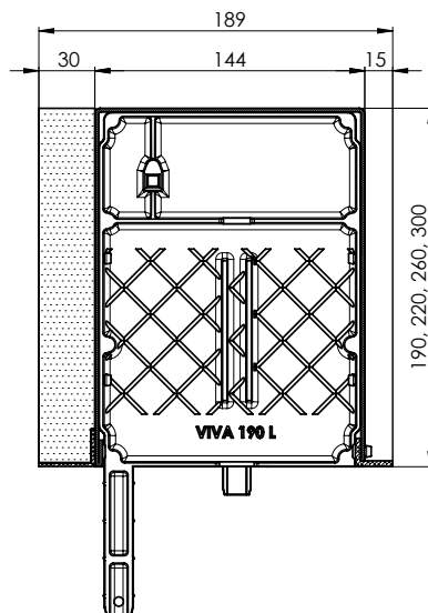
Schnitt durch den Unterputz-Kasten VIVA 190 x 189 x 2L x STY30 220 x 189 x 2L x STY30 260 x 189 x 2L x STY30 300 x 189 x 2L x STY30
