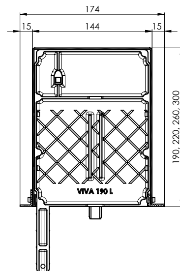
Schnitt durch den Unterputz-Kasten VIVA 190 x 160L2b 220 x 160L2b 260 x 160L2b 300 x 160L2b
