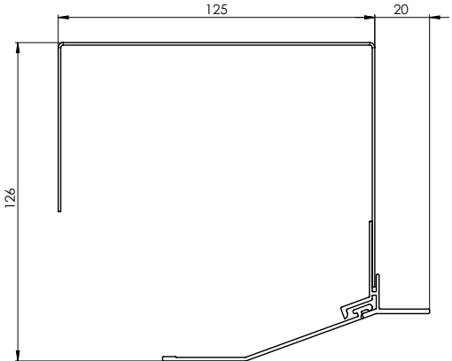
Box für Underputz-ausführung (PR0054 + PR0077 + PR0647)
