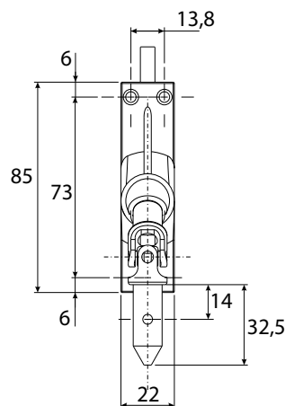
Durchföhrung 45°
