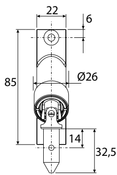
Durchföhrung 90°
