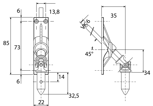
Durchführung 45°
