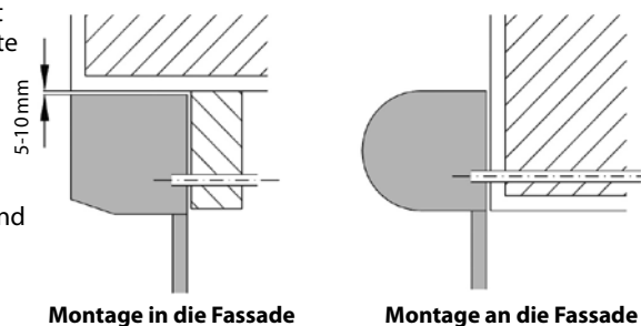
Montage in die Fassade
