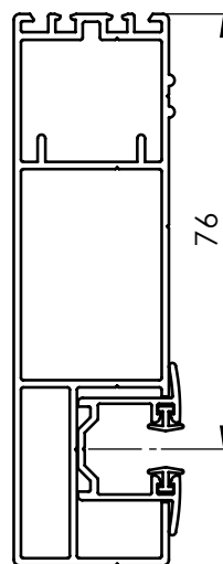
Größtmögliche Erweiterung des Grundprofils P 081
