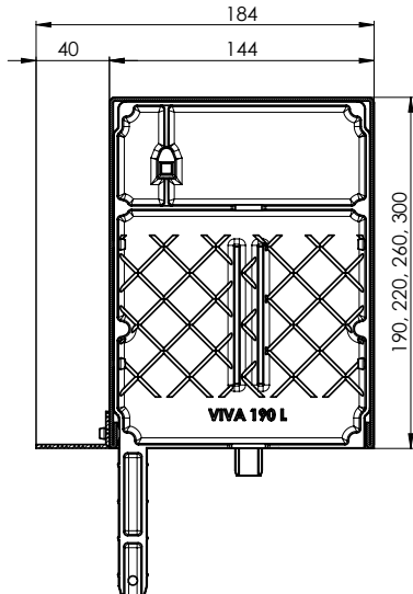
Schnitt durch den sichtbaren Kasten VIVA + P 020/04, P 080/04, P 081/04 190x140b 220x140b 260x140b 300x140b
