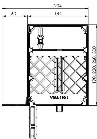
Schnitt durch den sichtbaren Kasten VIVA + P 020/06, P 080/06, P 081/06
