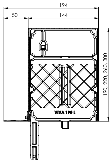
Schnitt durch den sichtbaren Kasten VIVA + P 020/05, P 080/05, P 081/05 190 x 140b 220 x 140b 260 x 140b 300 x 140b
