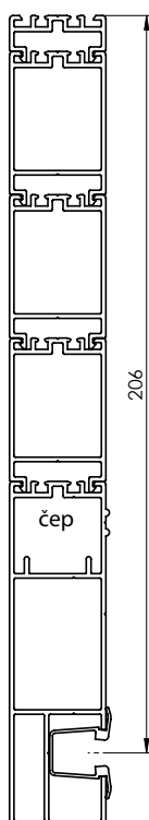
Größtmögliche Erweiterung des Grundprofils P 020
