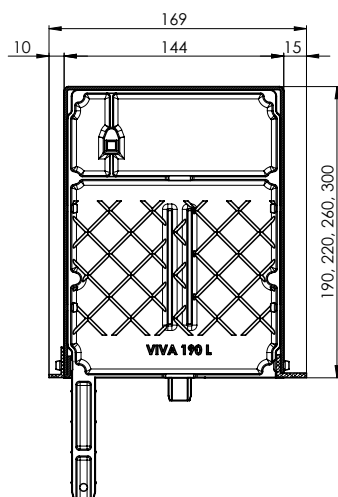
Schnitt durch den Unterputz-Kasten VIVA + P 020/01, P 080/01, P 081/01
