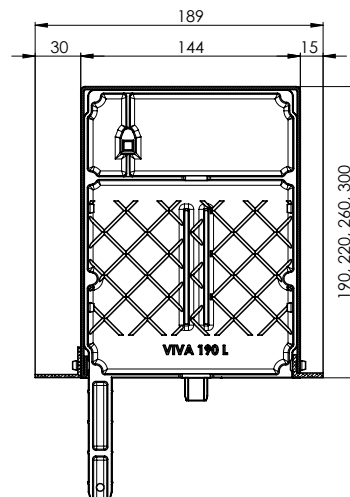
Schnitt durch den Unterputz-Kasten VIVA + P 020/03, P 080/03, P 081/03
