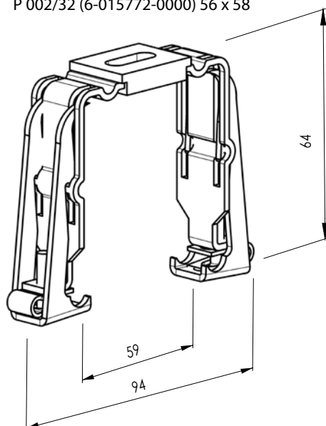
Oberschienenhalter mechanisch - Fe Click P 002/32 (6-015772-0000) 56 x 58
