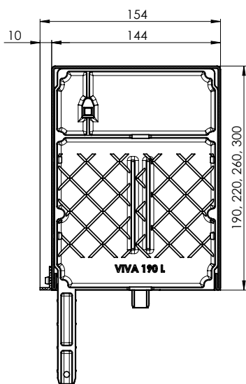
Schnitt durch den sichtbaren Kasten VIVA + P 020/01, P 080/01, P 081/01 190 x 140b 220 x 140b 260 x 140b 300 x 140b
