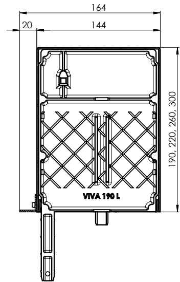
Schnitt durch den sichtbaren Kasten VIVA + P 020/02, P 080/02, P 081/02 190 x 140b 220 x 140b 260 x 140b 300 x 140b
