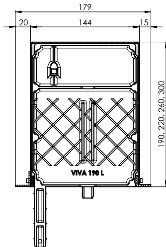
Schnitt durch den Unterputz-Kasten VIVA + P 020/02, P 080/02, P 081/02
