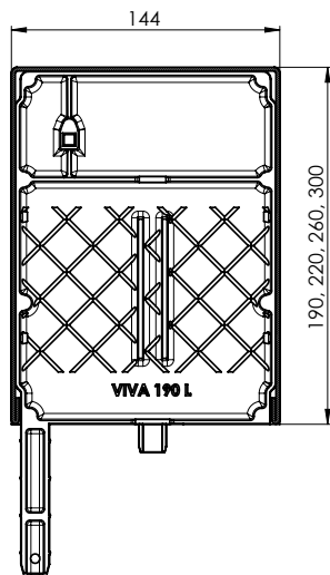
Schnitt durch den sichtbaren Kasten VIVA 190x140b 220x140b 260x140b 300x140b
