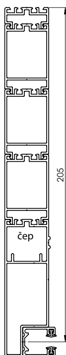
Größtmögliche Erweiterung des Grundprofils P 080
