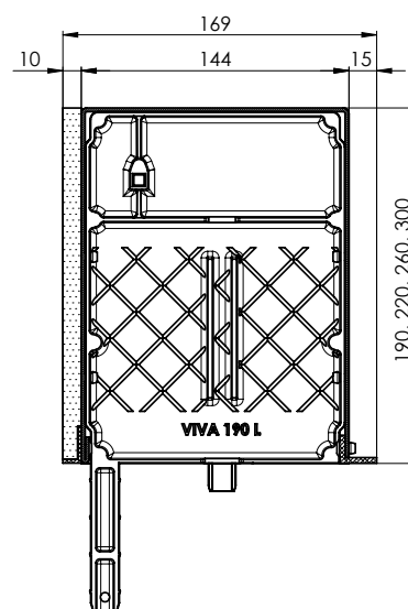
Schnitt durch den Unterputz-Kasten VIVA 190 x 169 x 2L x STY10 220 x 169 x 2L x STY10 260 x 169 x 2L x STY10 300 x 169 x 2L x STY10
