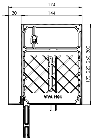
Schnitt durch den sichtbaren Kasten VIVA + P 020/03, P 080/03, P 081/03 190 x 140b 220 x 140b 260 x 140b 300 x 140b
