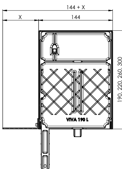
Schnitt durch den sichtbaren Kasten VIVA + P 020/07-20, P 080/07-20, P 081/07-20
